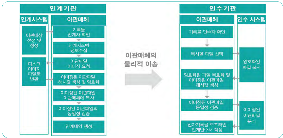
[이관매체를 사용한 전자기록물의 오프라인 이관 흐름도]
