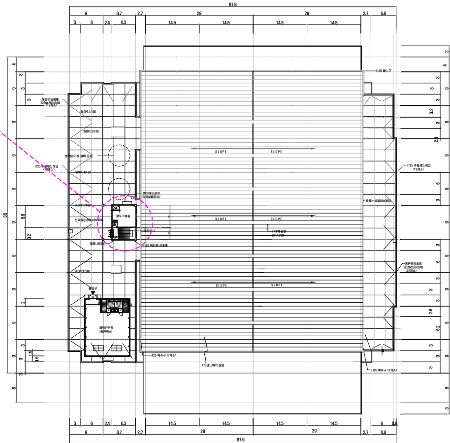
옥상층 평면도
